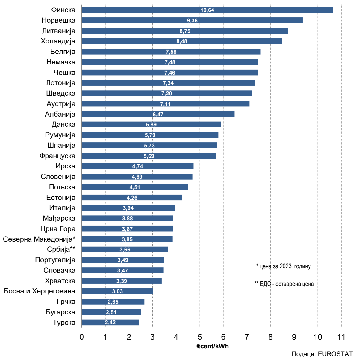
Слика 3-7: Цене приступа дистрибутивном систему у европским државама за домаћинство у 2024. години
