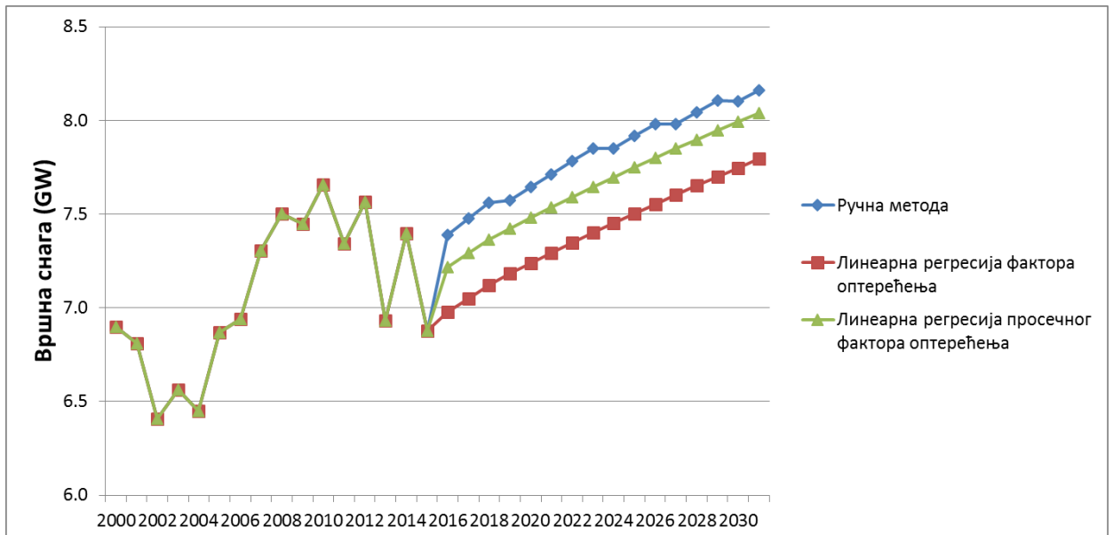
Слика 2.9 – Прогноза вршне снаге Републике Србије за сценарио средњег раста за више метода прогнозе фактора оптерећења
