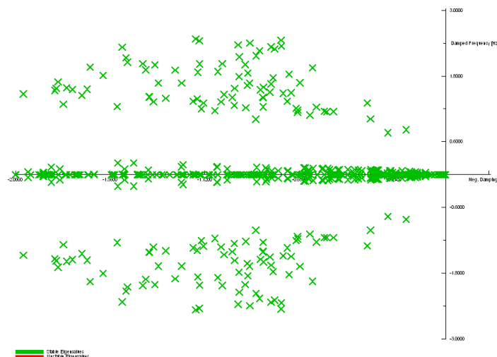
Слика 7: Корени карактеристичне једначине ЕЕС Србије за режим зимског максимума 2019. године
