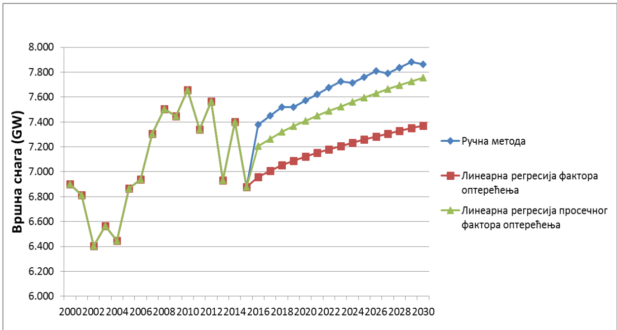
Слика 2.8 – Прогноза вршне снаге Републике Србије за сценарио нижег раста за више метода прогнозе фактора оптерећења
