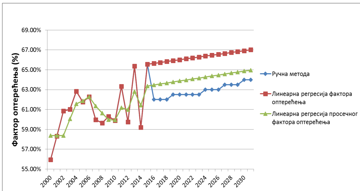
Слика 2.7 – Прогноза фактора оптерећења ЕЕС Републике Србије до 2031. године
