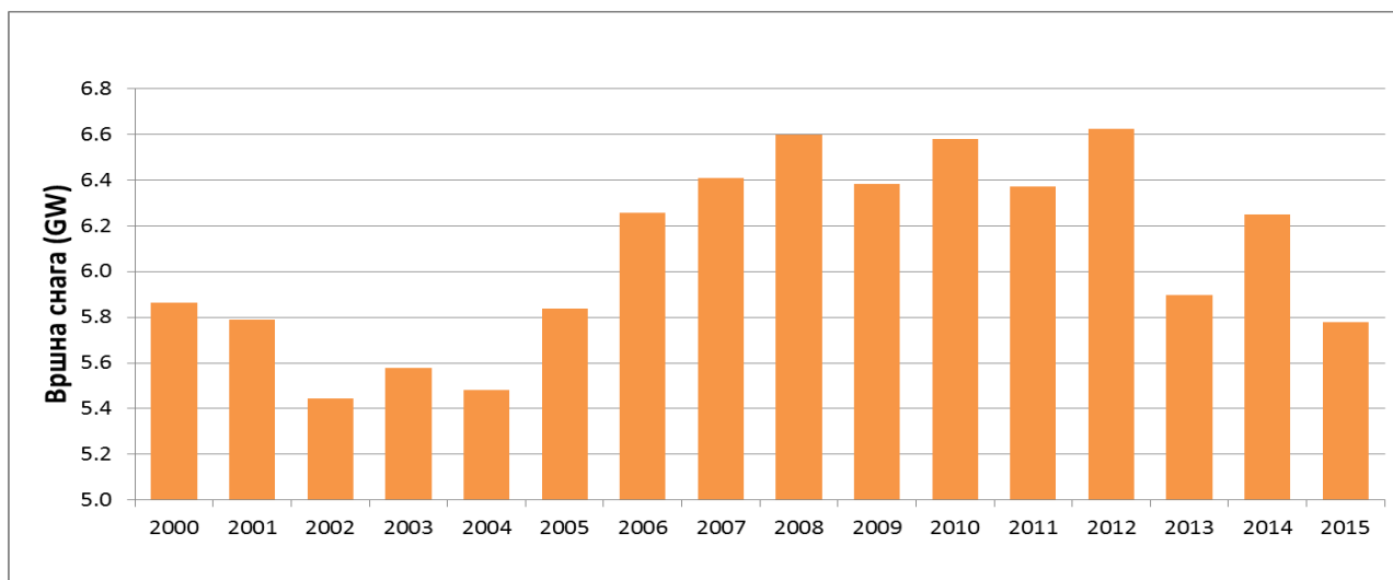
Слика 2.17: Остварене вредности вршне снаге ЕЕС Републике Србије без Косова и Метохије за период 2000. – 2015. године
