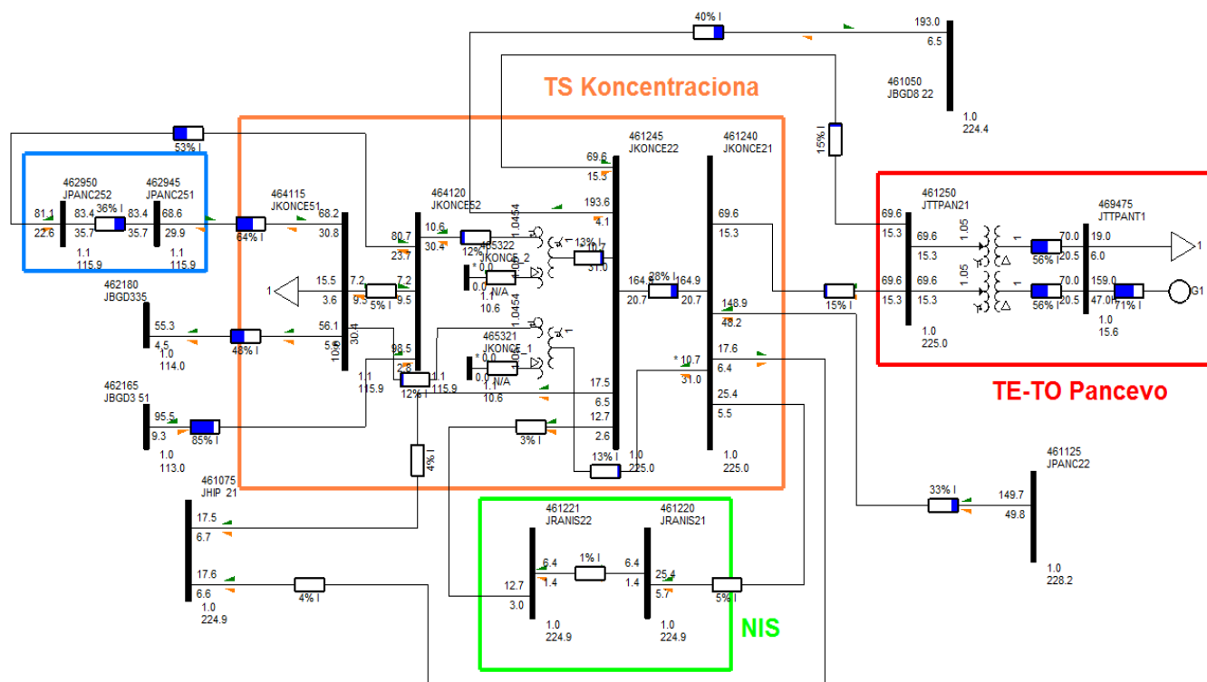
Слика 1.4: Анализа токова снага и напонских прилика у ТС Панчево 7 у зимског максимума у 2026.години
